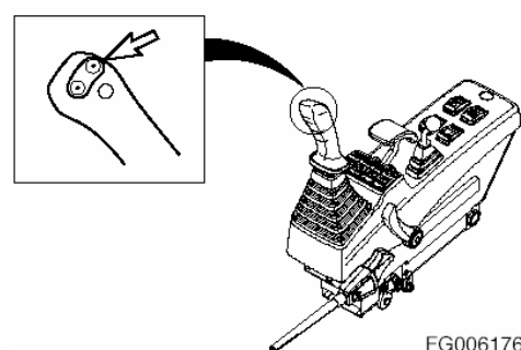
Figura 99 PALANCA DE MANDO IZQUIERDA (JOYSTICK)
