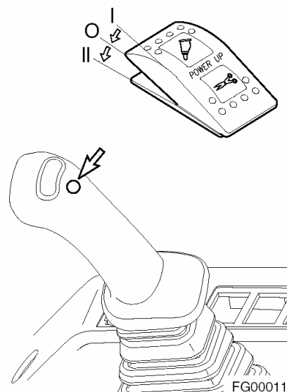
Figura 53 PALANCA DE MANDO DERECHA (JOYSTICK)
